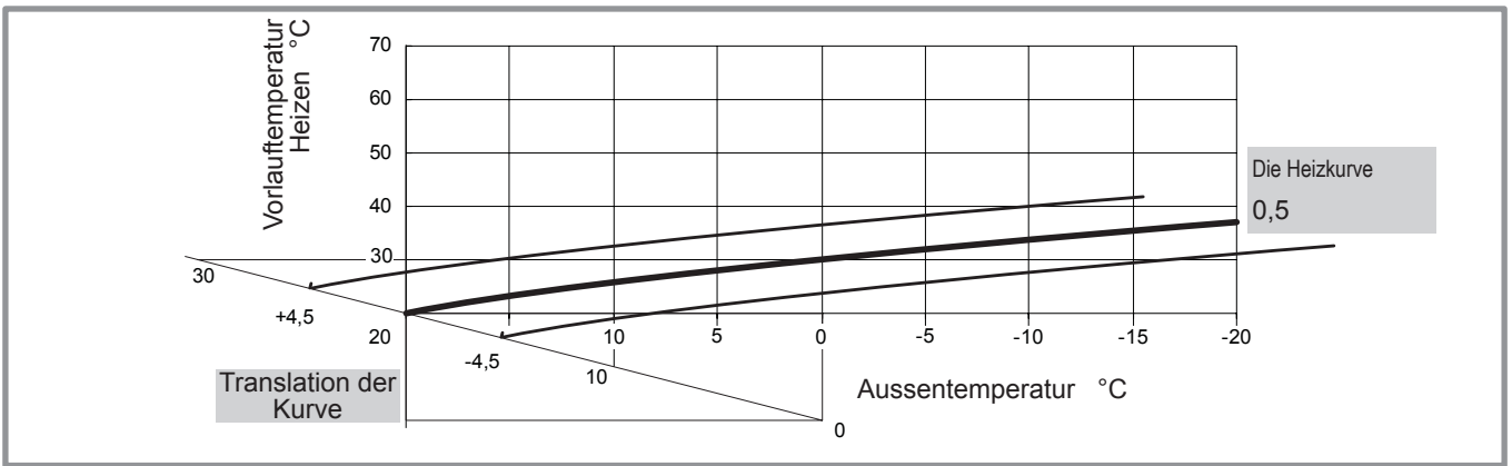
Abbildung 47 - Verschiebung der Heizkurve (Zeile 721)
