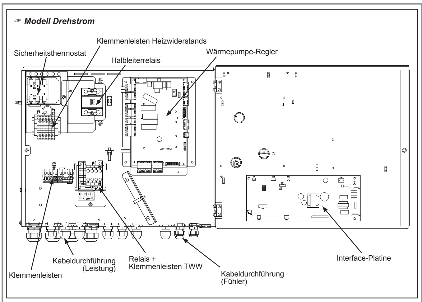
Abbildung 41 - Zugang zum Schaltkasten des Hydraulikmoduls und Beschreibung
