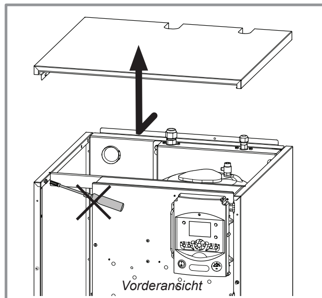
Abbildung 15 - Abnehmen des Deckels
