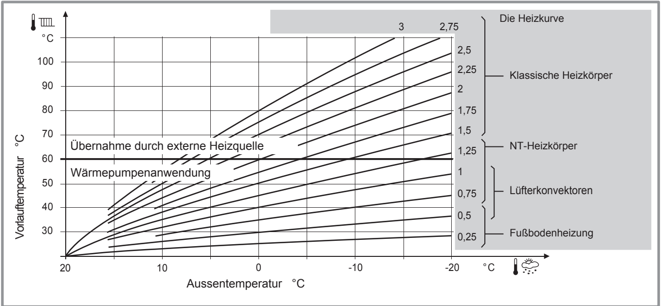
Abbildung 46 - Gefälle der Heizkurve (Zeile 720)
