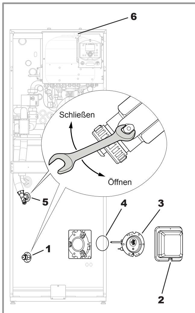
Abbildung 56 - Entleeren des Hydraulikmoduls und/oder Entleeren des WW-Speichers
