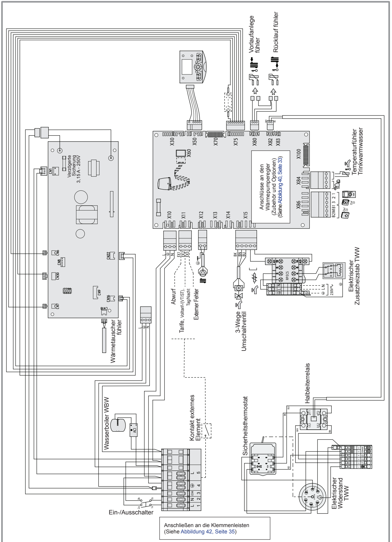
Abbildung 52 - Elektrische Verkabelung Hydraulikmodul (Außer Installateuranschlüsse)
