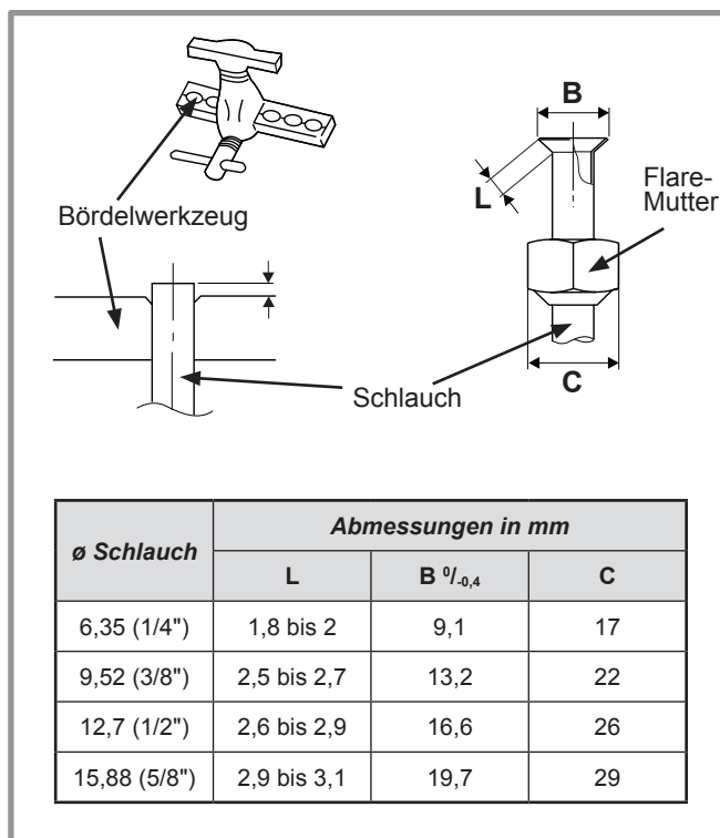
Abbildung 16 - Aufweiten für Flare-Verbindung
