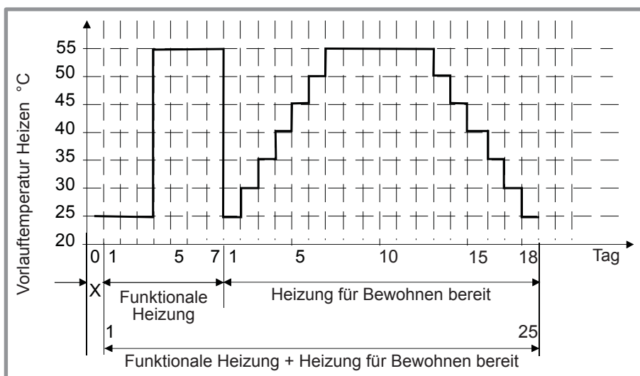
Abbildung 49 - Diagramm der Bodentrockenprogramme
