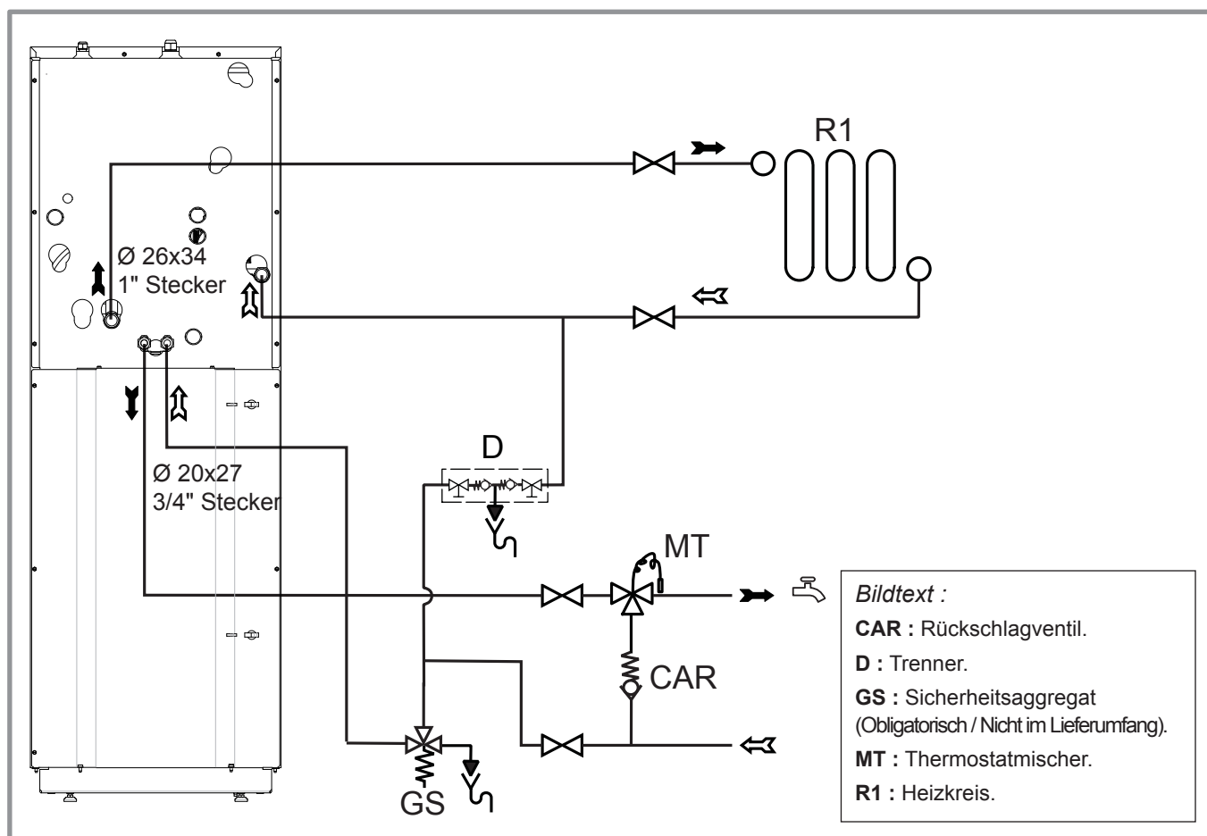
Abbildung 22 - Hydraulikwirkbild
