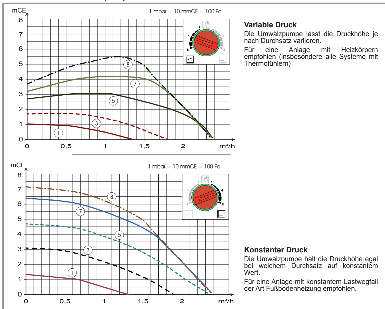
Abbildung 28 - Vorh. Ext. Pressung und Volumenstrom
