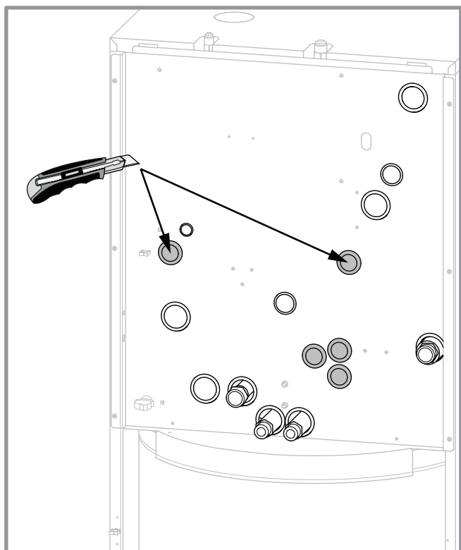
Abbildung 39 - Kabeldurchführung auf der Hinterseite der Inneneinheit
