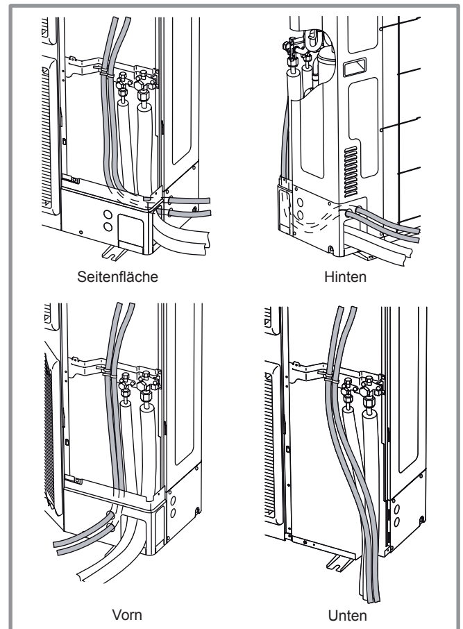
Abbildung 38 - Durchführungen der Kabel und der Kühlleitungen der Außeneinheit Drehstrom
