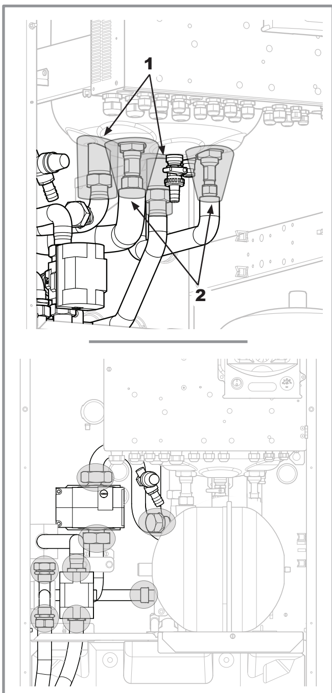
Abbildung 27 - Wärmeisolierung
