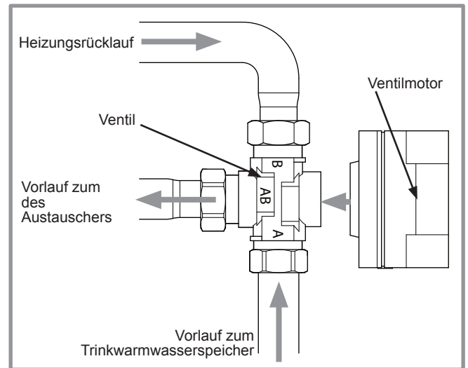
Abbildung 57 - Montage des Richtungsventils
