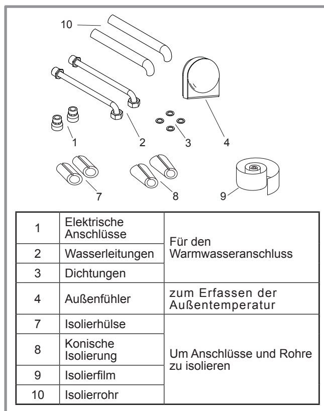
Abbildung 10 - Mit der Hydraulikmodul geliefertes Zubehör
