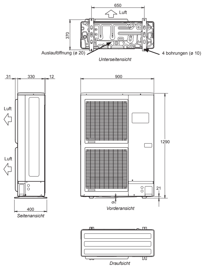
Abbildung 1 - Abmessungen in mm
