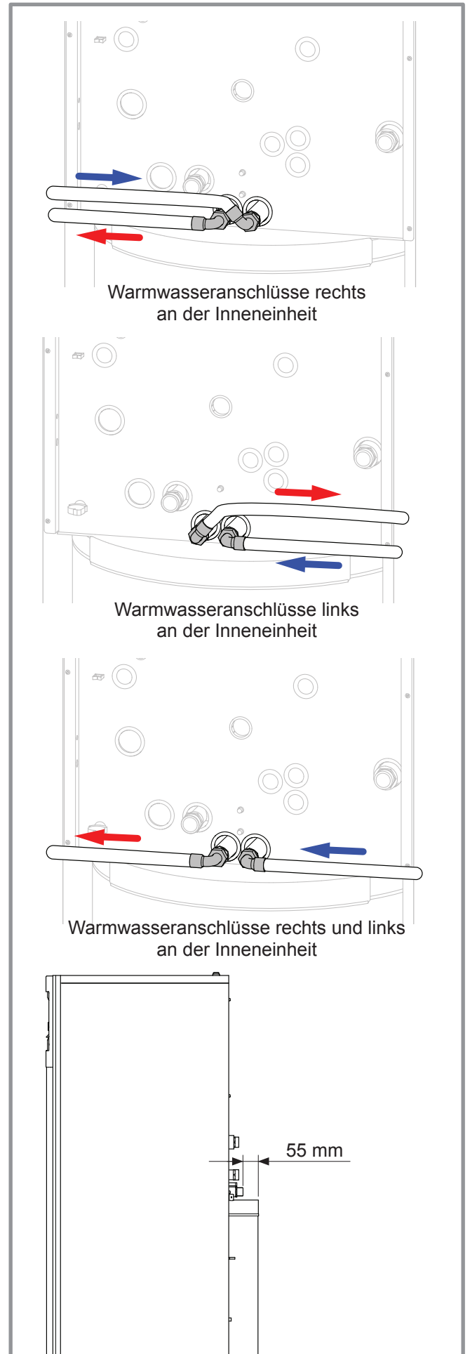
Abbildung 24 - Warmwasseranschlüsse
