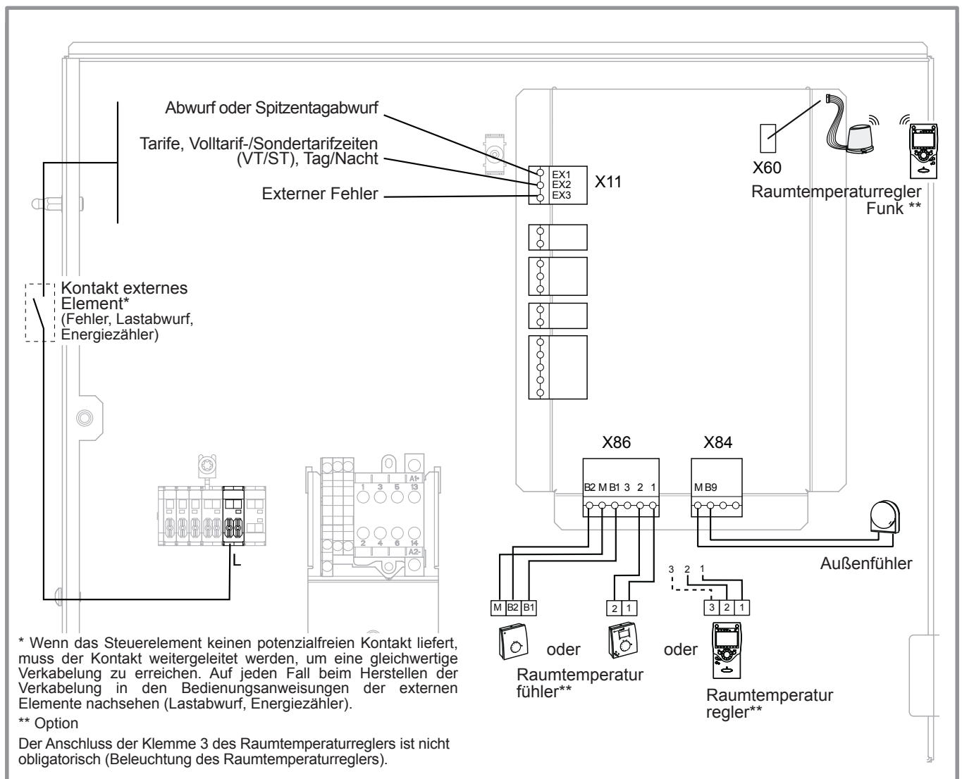
Abbildung 40 - Anschlüsse an den Wärmepumperegler (Zubehör und Optionen)
