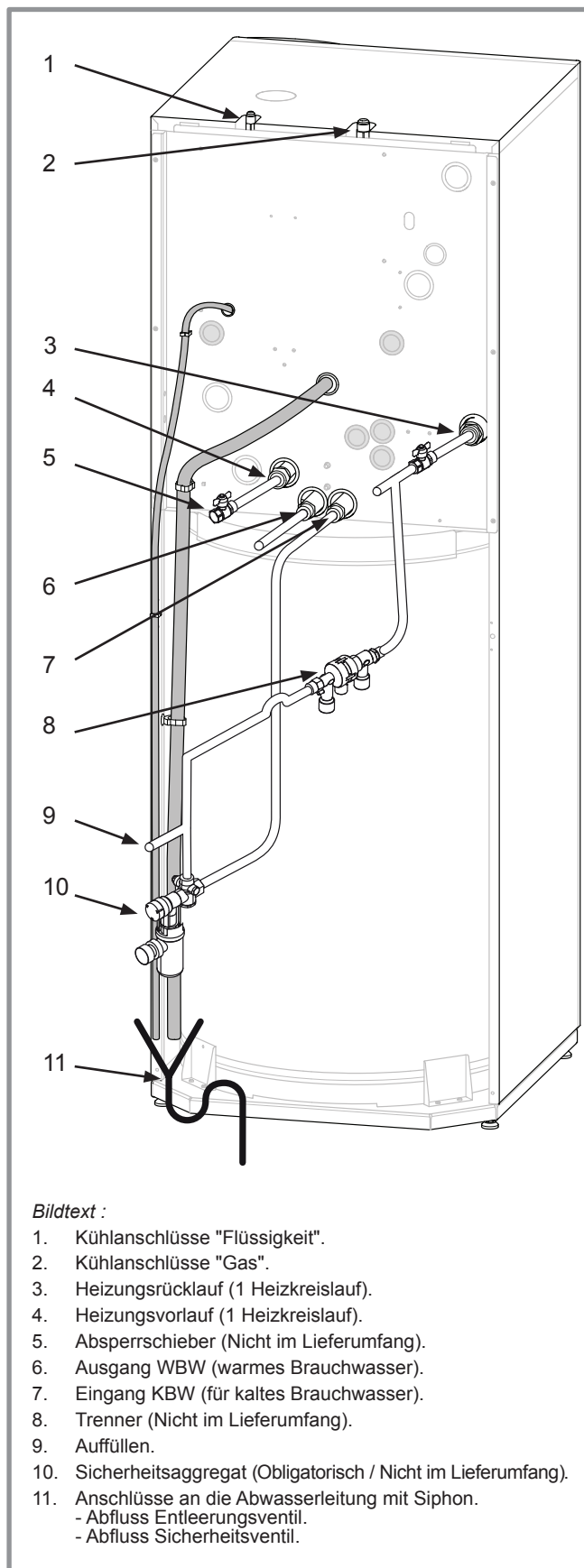
Abbildung 25 - Anschlüsse
