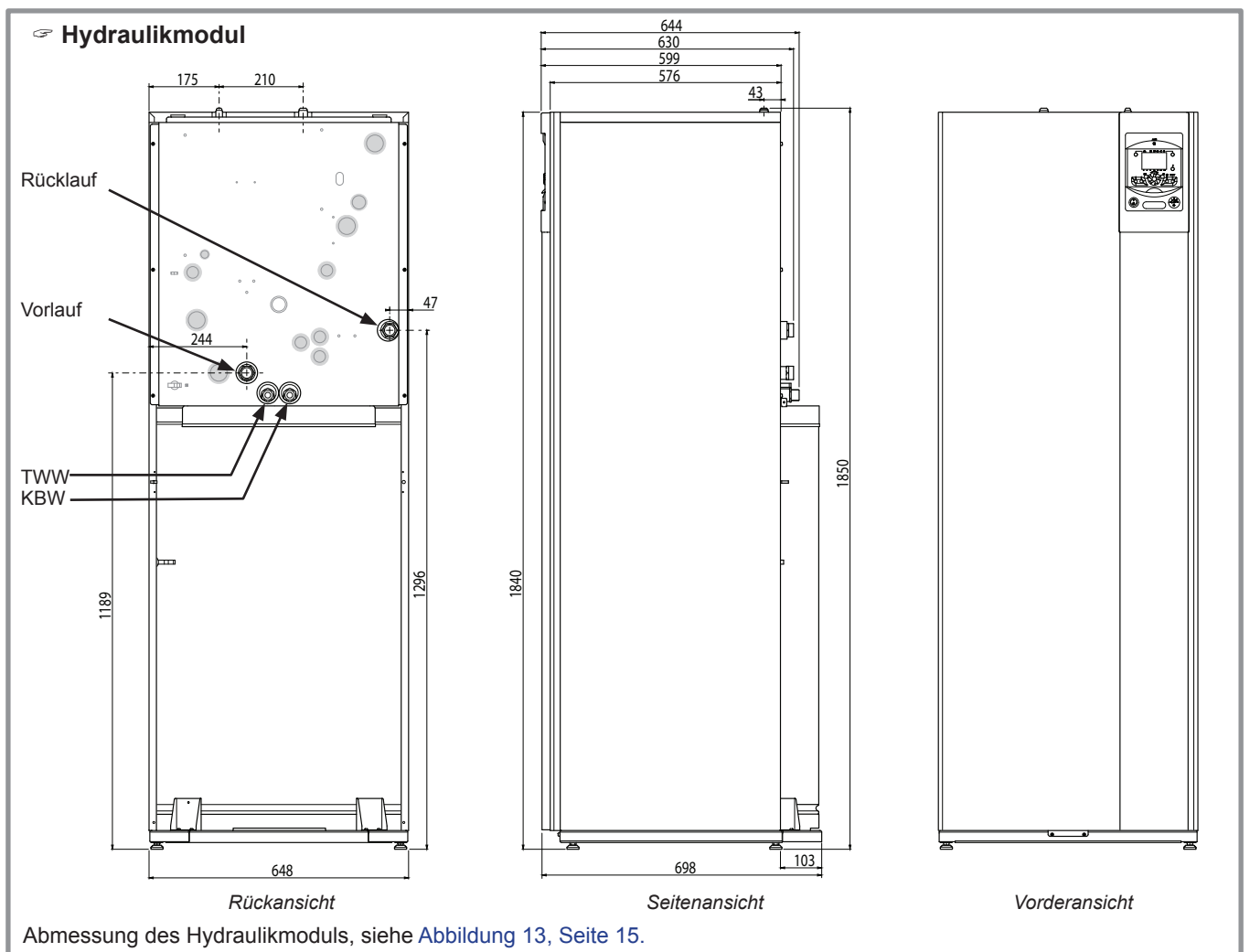
Abbildung 2 - Abmessungen in mm
